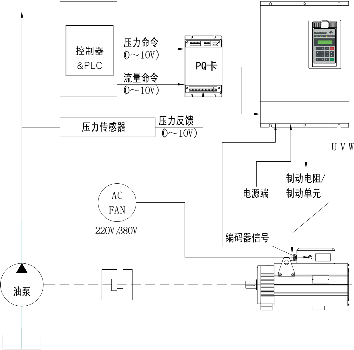
5.5 电液伺服系统图 2
