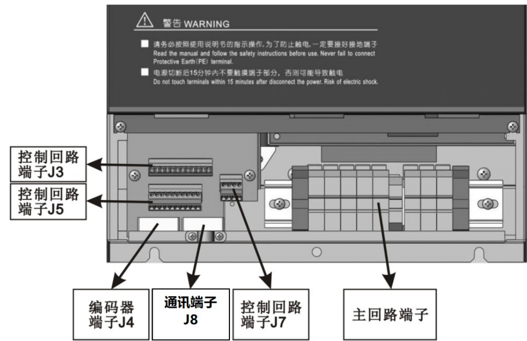
图 5.3.2 驱动器接口端子示意图（适合于 22~75kW）
